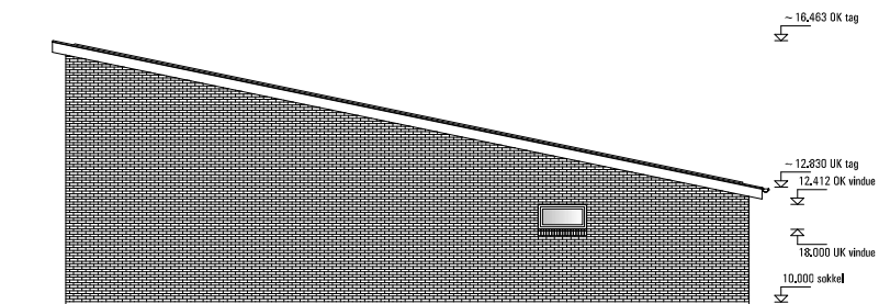
FACADE MOD NORD-VEST
