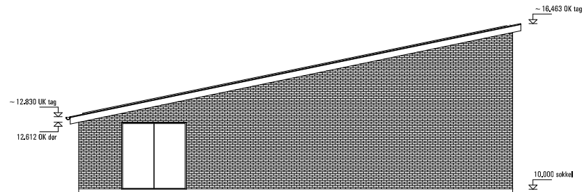
FACADE MOD SYD-ØST
